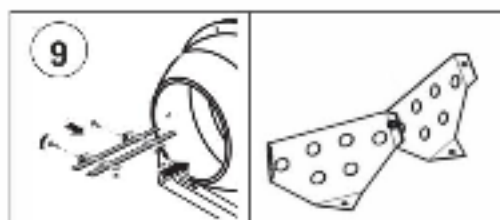
Болт M8x20 x2 Гайка M8 x2 Шайба d8 x2
